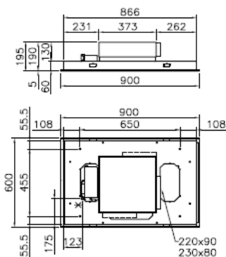
SALIERI 90 (21Kg) HERA 90 (21Kg)
