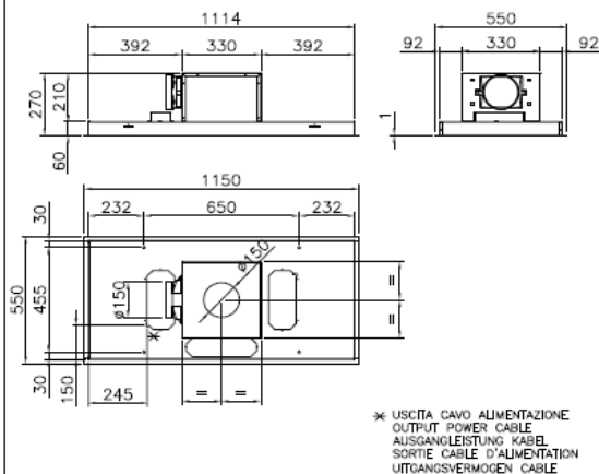
FENICE 120 CON MOTORE (22kg)
