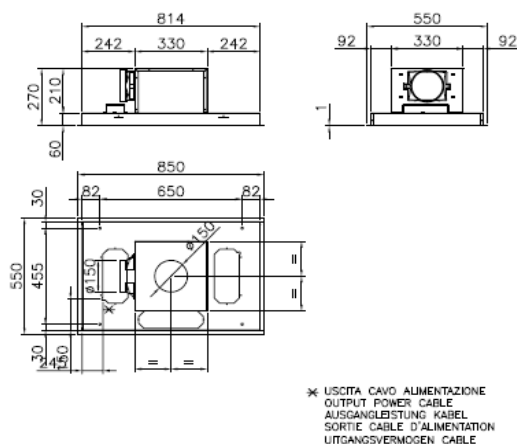
FENICE 90 CON MOTORE (16kg)
