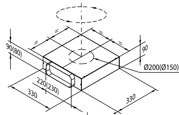
KIT SENZA MOTORE
