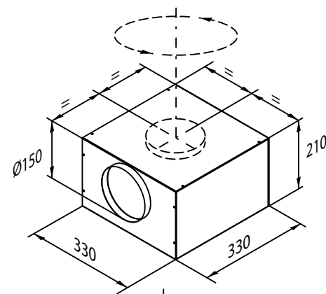
KIT MOTORE H850
