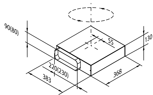
KIT MOTORE E1300
